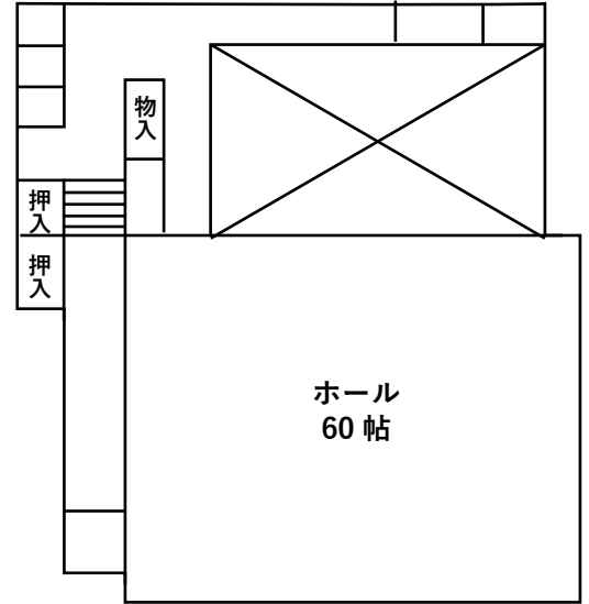
別館 1階
